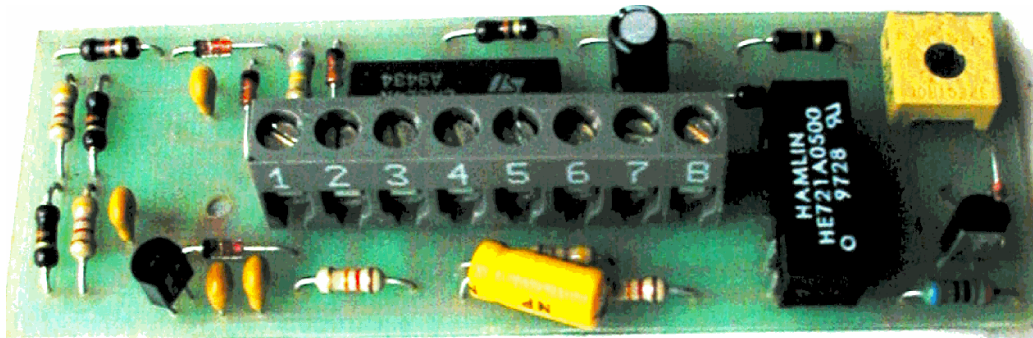
Abschaltbare Linienverzögerung (12K0hm)
