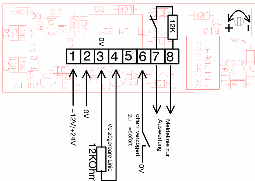
Abschaltbare Linienverzögerung (12K0hm)
